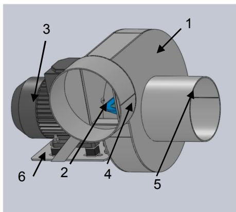
Рис. 1 Конструкция вентилятора
