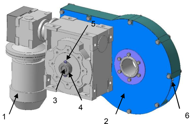
Рис.3 Привод колосника для котлов мощностью 600 – 1000 кВт
